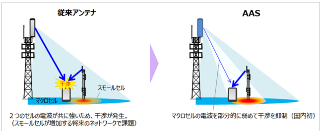
(図3)指向性制御技術による通信品質改善のイメージ
